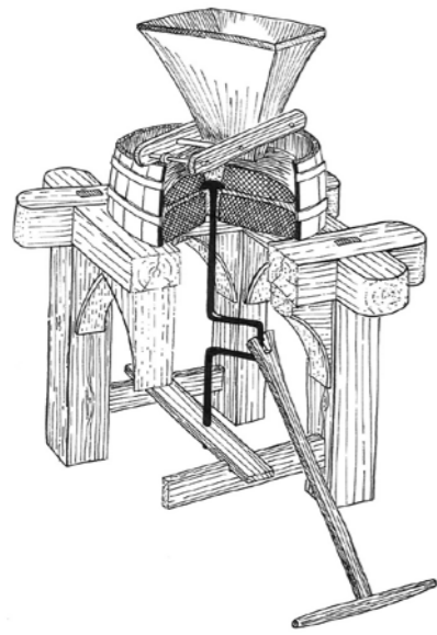
Tekening met doorsnede van een handgrutmolen zoals Roel Schipper ook zal hebben gebruikt
