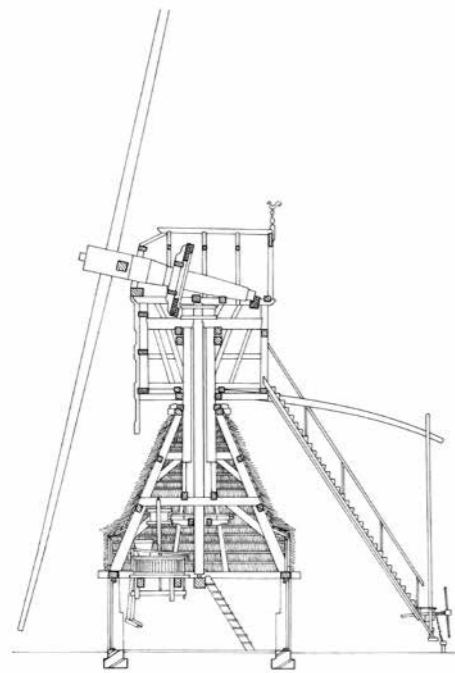
Doorsnede van een wipkorenmolen
